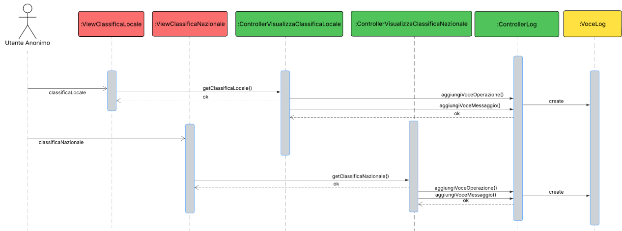
Figura 40: Diagramma di interazione relativo alle Classifiche
