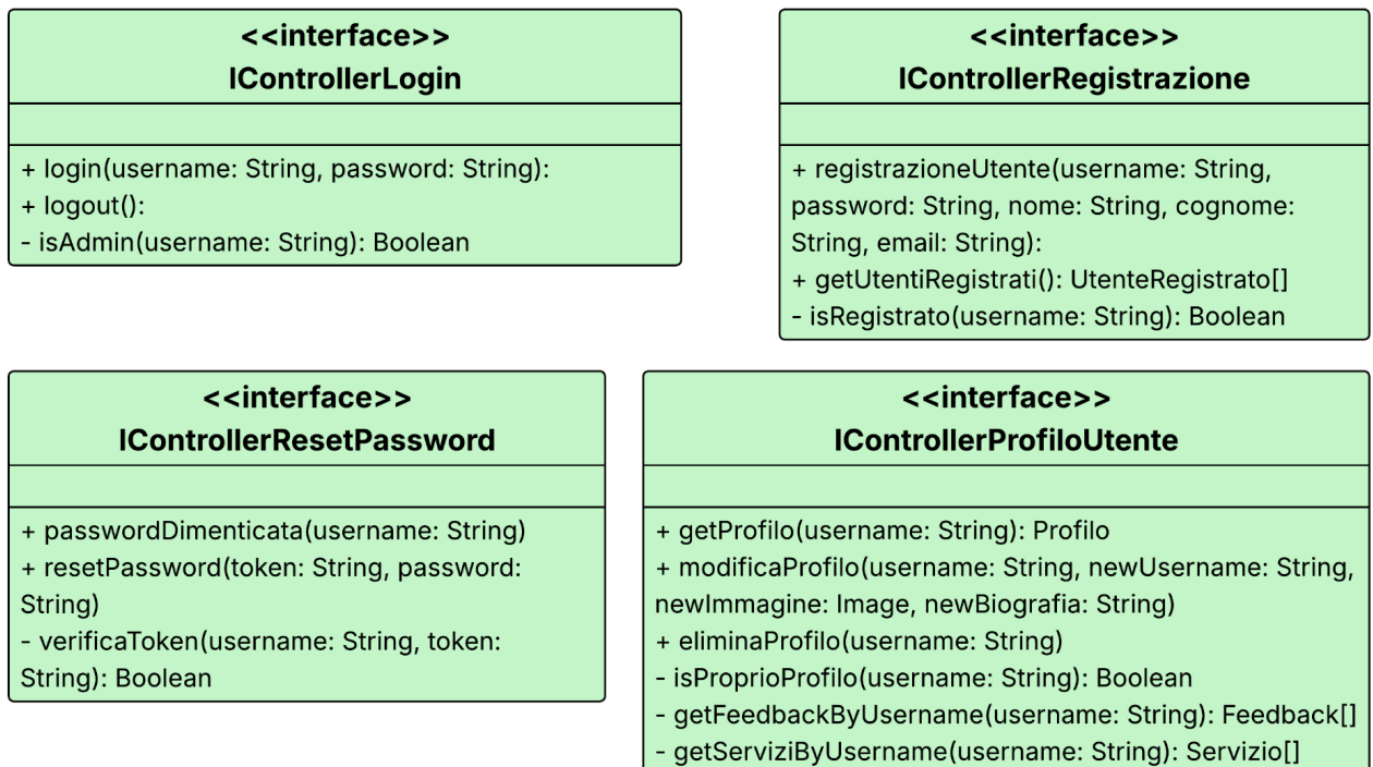
Figura 16: Interfacce dei controller relativi all'Utente e al Profilo
