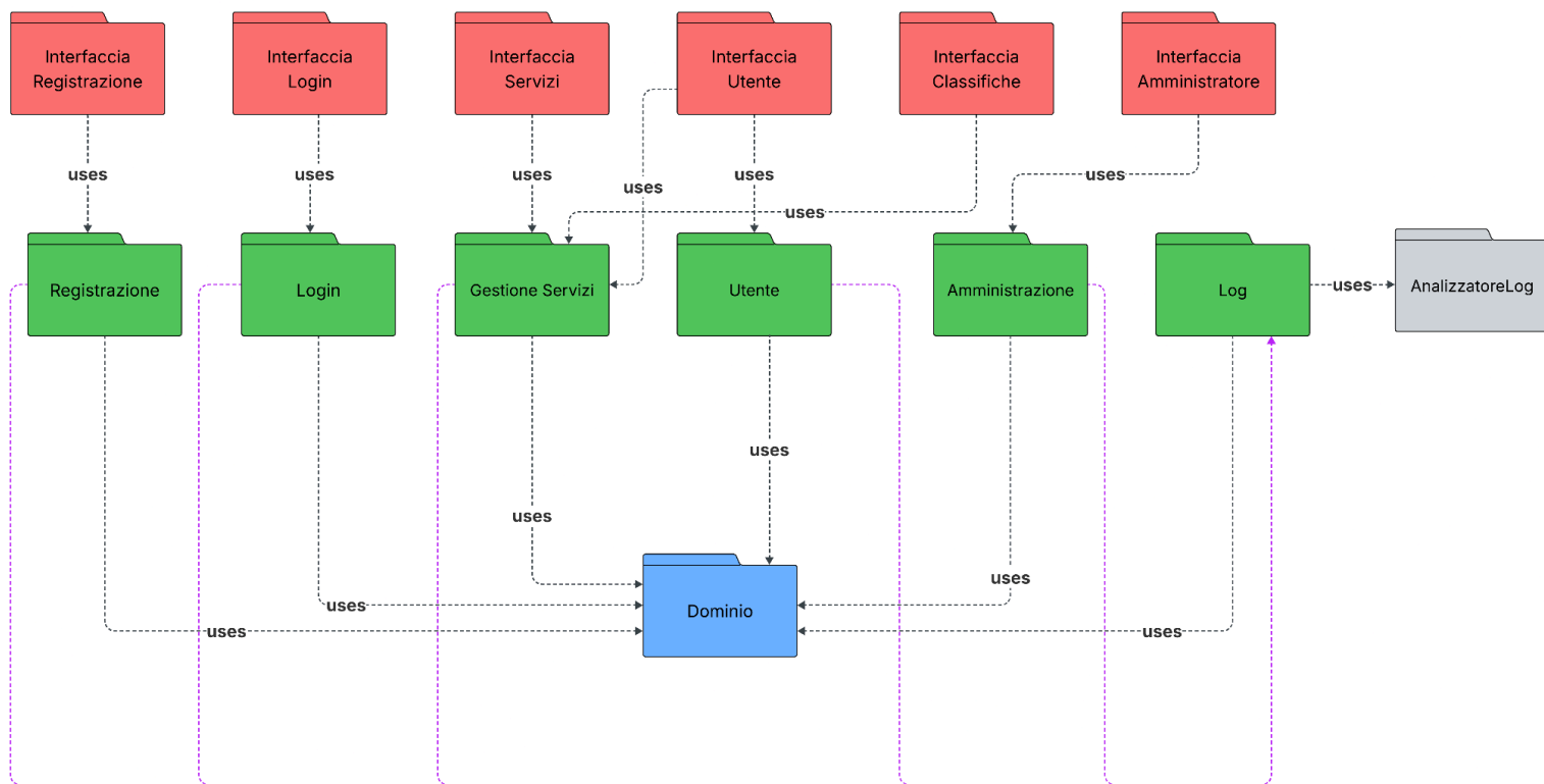
Figura 5: Diagramma dei package
