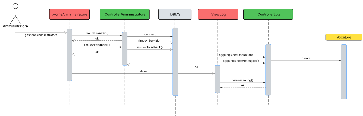
Figura 37: Diagramma di interazione relativo all'Amministrazione
