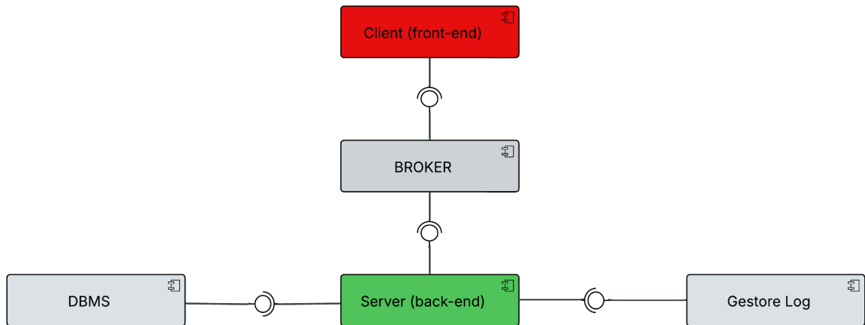
Figura 15: Diagramma dei Componenti
