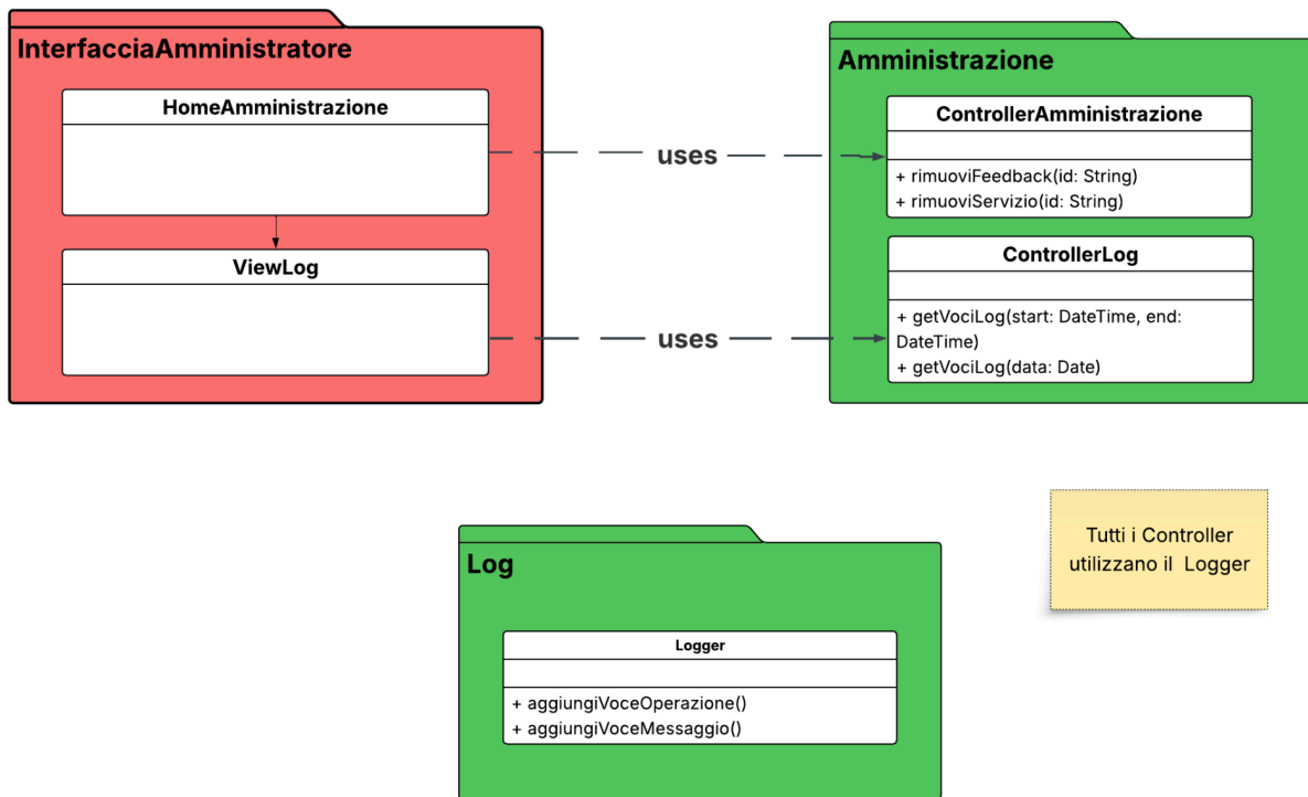
Figura 7: Diagramma delle classi relativo all'Amministratore e al Log
