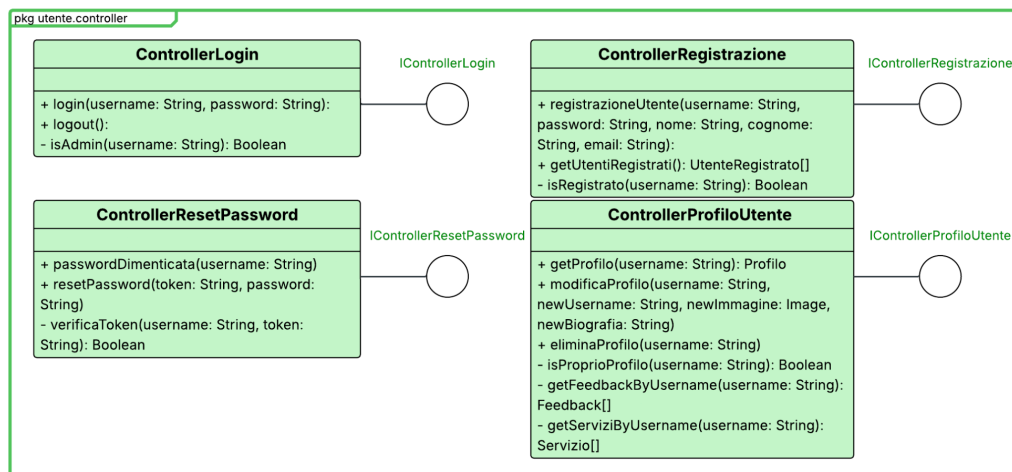
Figura 21: Struttura dei controller relativi alla gestione degli Utenti
