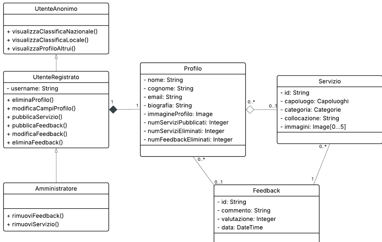
Figura 1: Relazione tra Utenti, i Servizi e i Feedback
