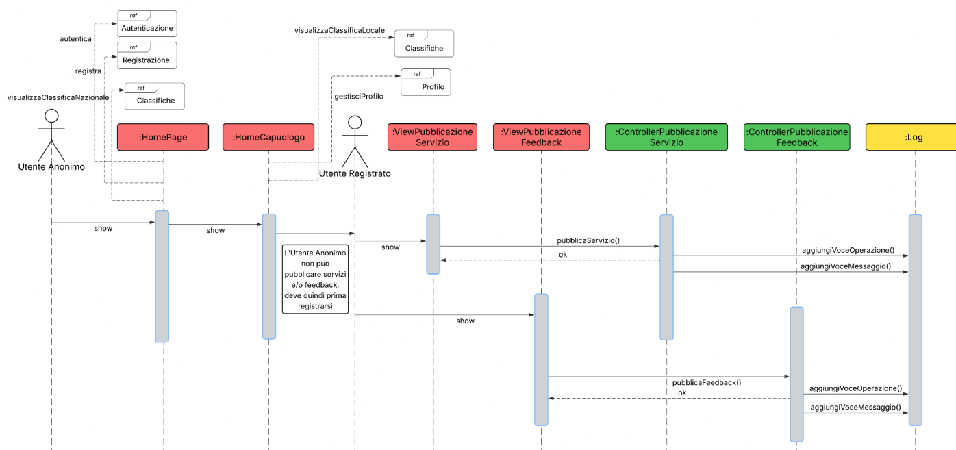
Figura 11: Diagramma di sequenza relativo ai Servizi e i Feedback
