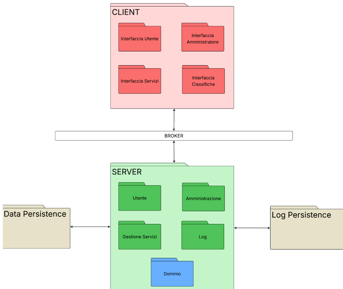
Figura 14: Diagramma dei Package
