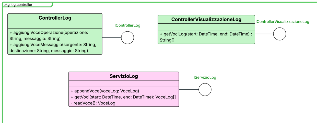
Figura 26: Struttura dei controller relativi alla gestione dei Log
