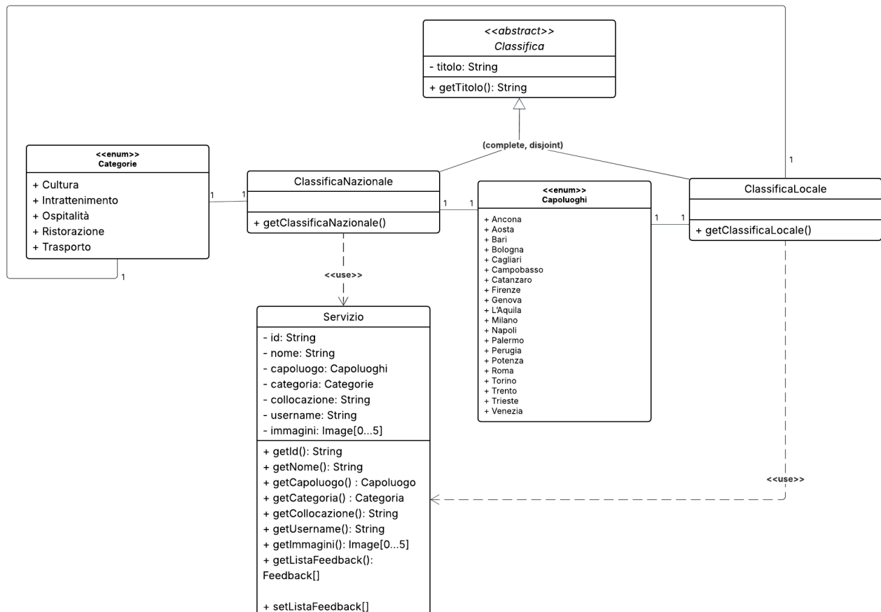
Figura 23: Diagramma di Dettaglio del dominio delle Classifiche
