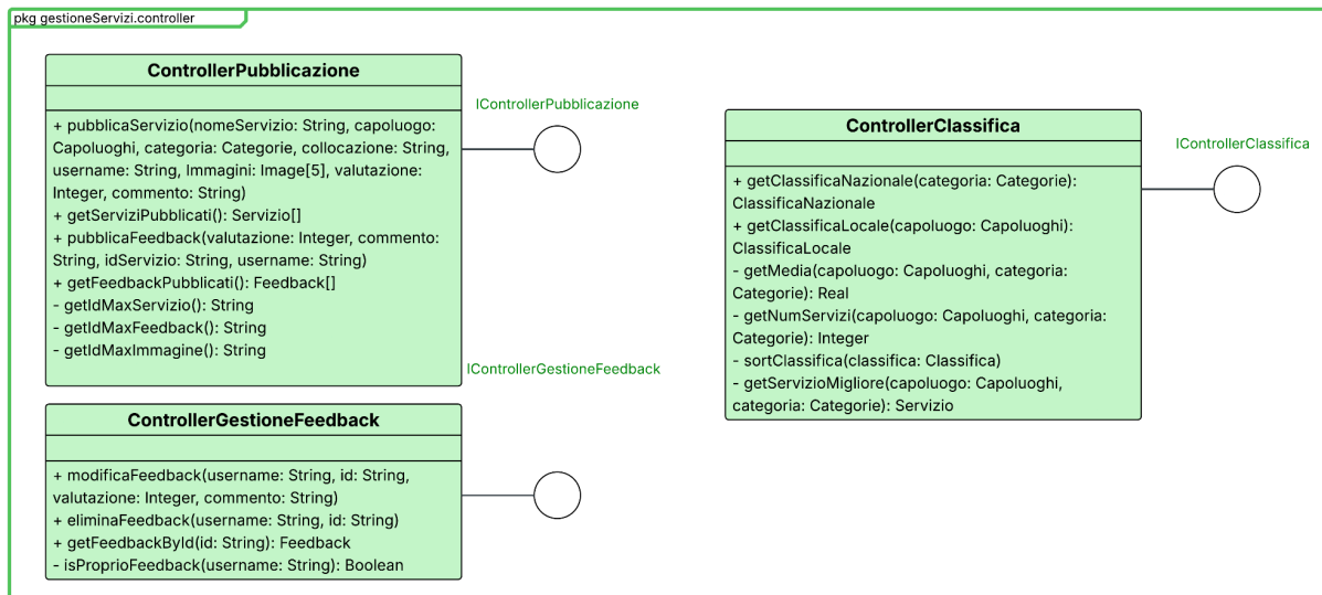
Figura 24: Struttura dei controller relativi alla gestione dei Servizi e dei Feedback
