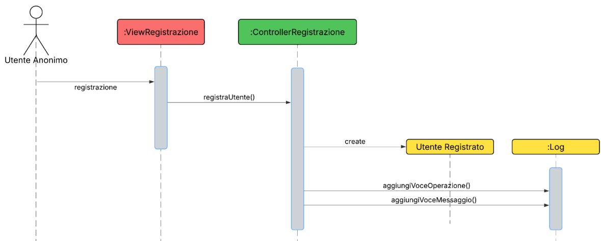
Figura 8: Diagramma di sequenza relativo alla Registrazione
