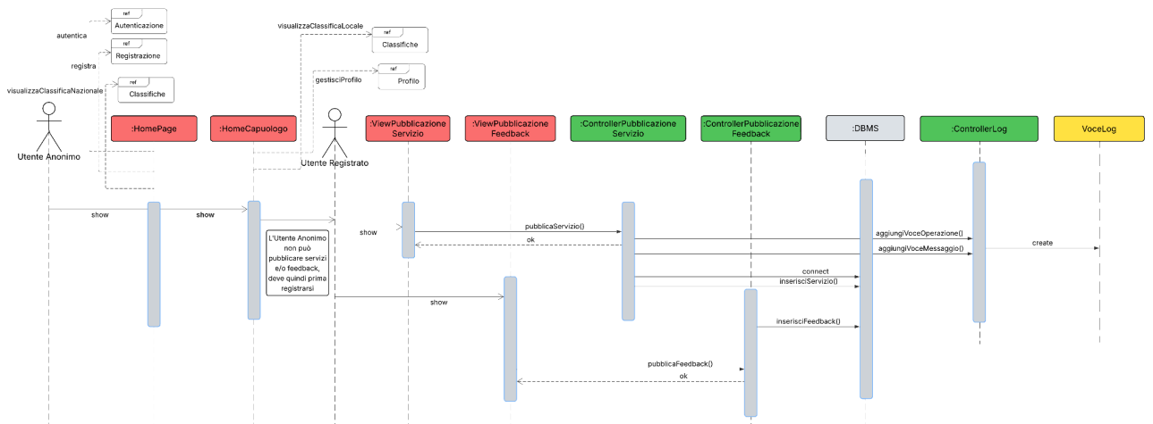
Figura 39: Diagramma di interazione relativo ai Servizi
