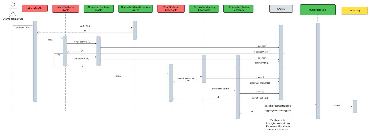
Figura 38: Diagramma di interazione relativo al Profilo
