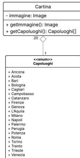
Figura 27: Diagramma di Dettaglio del dominio relativo alla Cartina
