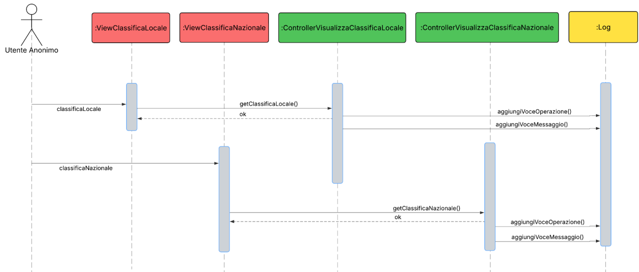
Figura 12: Diagramma di sequenza relativo alle Classifiche
