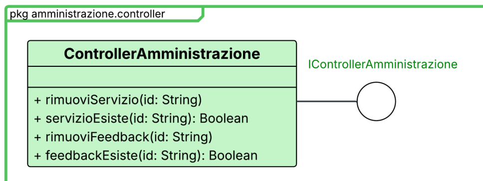
Figura 22: Struttura dei controller relativi alla gestione dell'Amministratore
