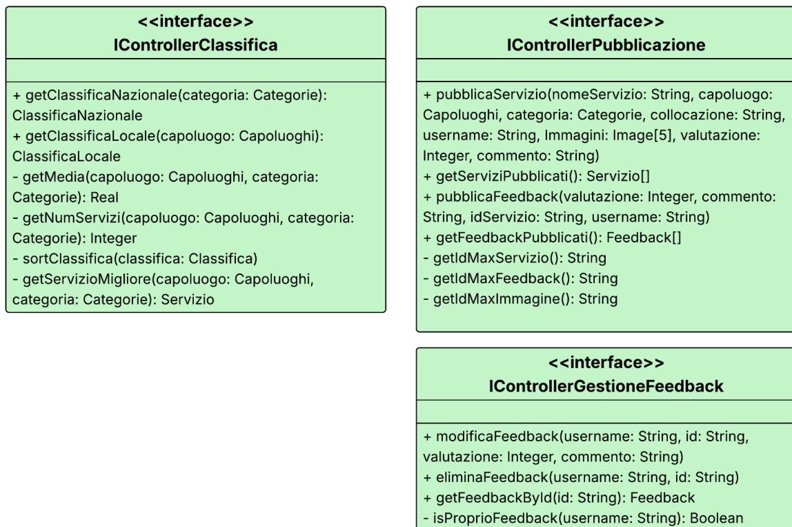
Figura 17: Interfacce dei controller relativi alle Classifiche e ai Servizi
