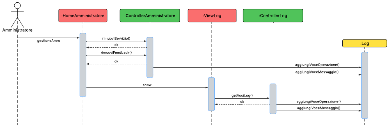
Figura 10: Diagramma di sequenza relativo all'Amministratore
