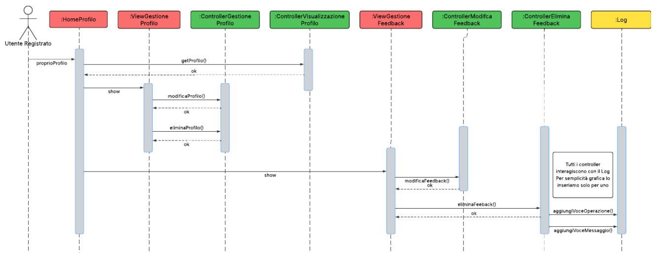
Figura 13: Diagramma di sequenza relativo al Profilo
